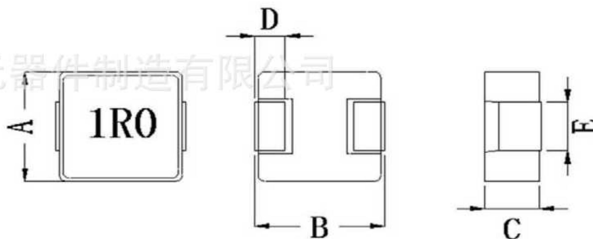
GCHR/GCHR一体成型电感器 图示和尺寸：（单位mm）
